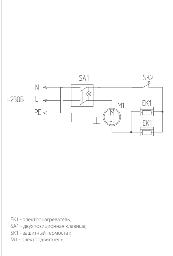
Подключение BHC-L05S02-S
