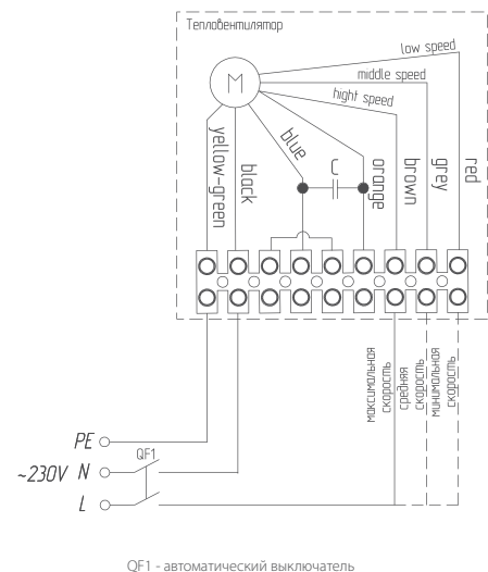
Тепловентилятор W2-S/W3-S к автоматическому выключателю*
