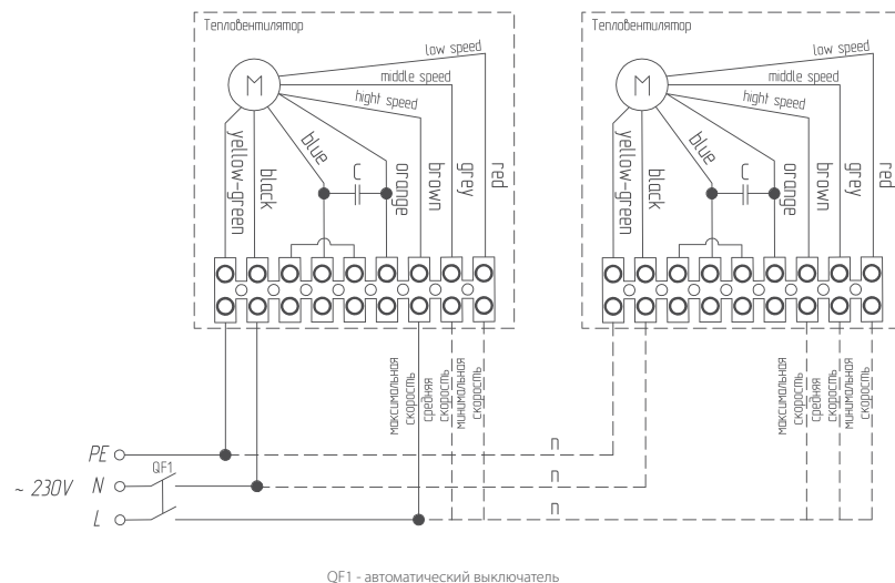
Групповое подключение тепловентиляторов W2-S/W3-S к автоматическому выключателю*
