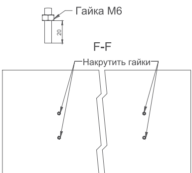
Расположение монтажных кронштейнов для горизонтальной установки на резьбовые шпильки
