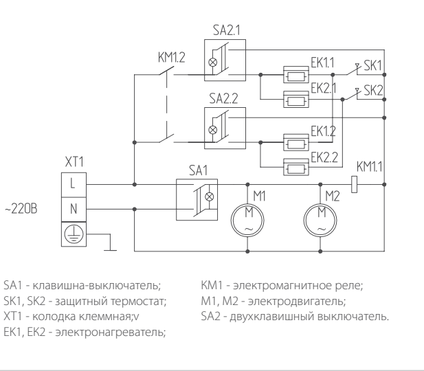
Подключение BHC-L08-S05-M
