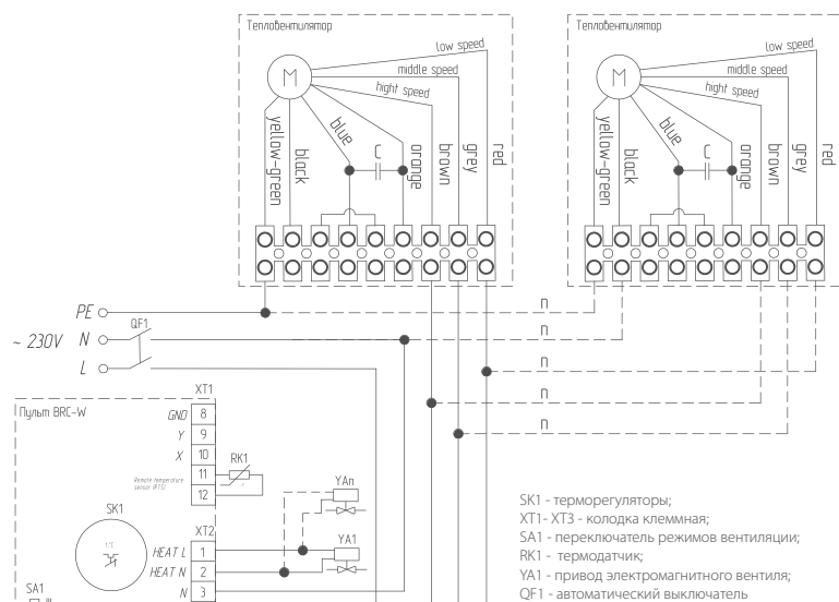
Групповое подключение тепловентиляторов W2-S/W3-S к пульту BRC-W
