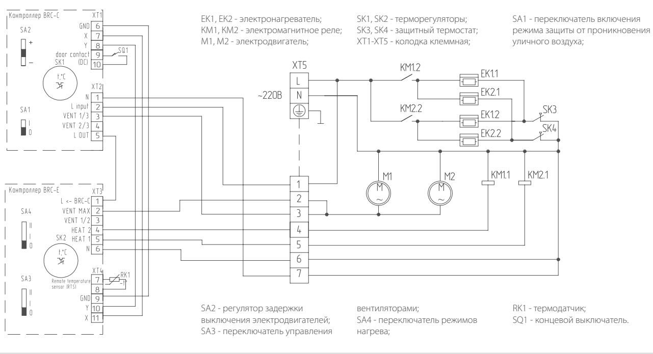
Групповое подключение BHC-L10-S06 (-M) к пульту BRC-E и BRC-C
