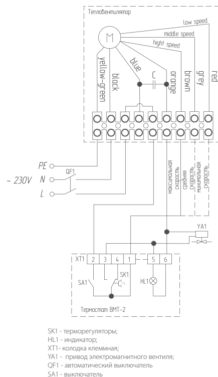
Тепловентилятор W2-S/W3-S к термостату BMT-2
