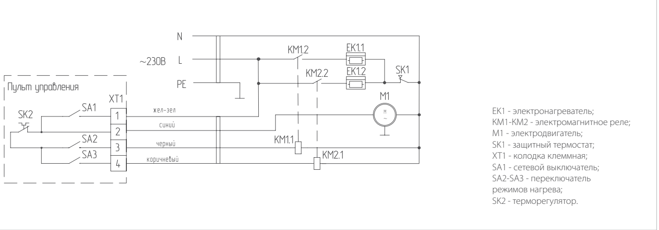
Подключение BHC-L11S06-SP
