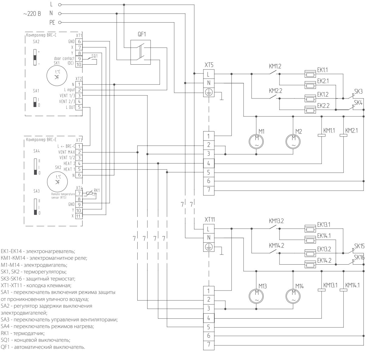
Групповое подключение BHC-L10-S06 (-M) к пульту BRC-E и BRC-C
