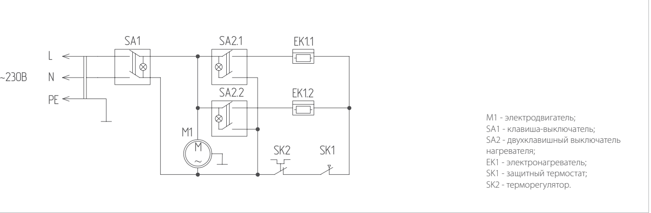
Подключение BHC-L09S03-SP
