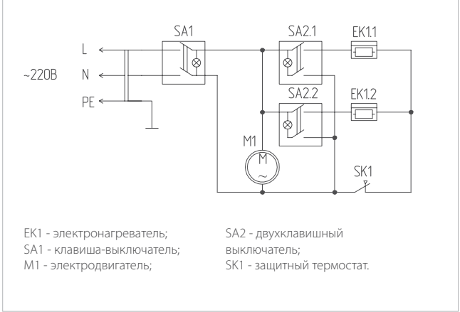
Подключение BHC-L06-S03
