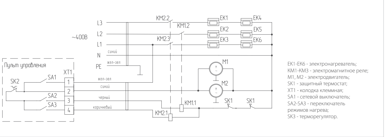
Подключение BHC-L15S09-SP
