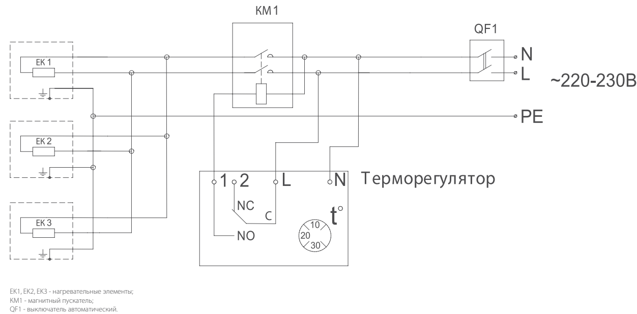
Схема электрическая принципиальная инфракрасных обогревателей BIH-S2-0.3 и BIH-S2-0.6 при групповом подключении к электрической сети, с использованием магнитного пускателя.
