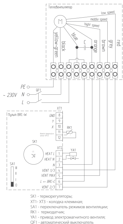
Тепловентилятор W2-S/W3-S к автоматическому выключателю*
