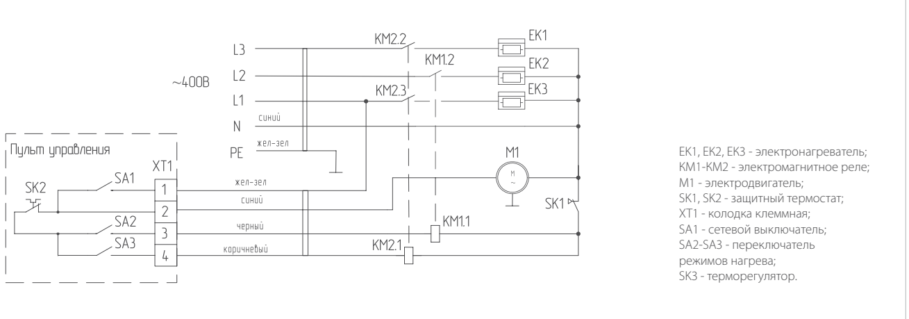
Подключение BHC-L15S09-SP
