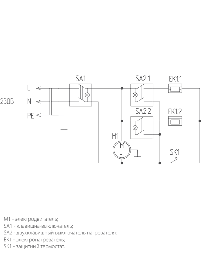
Подключение BHC-L06S03-S
