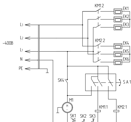
Схема коммутации переключателя
