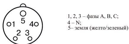
Рис.5 Схема контактов на вилке
